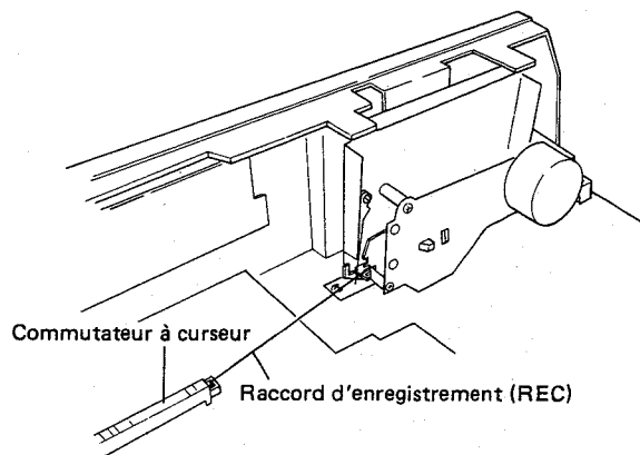
Fig. 10-3 Réglage et vérification du raccord d'enregistrement (REC)
