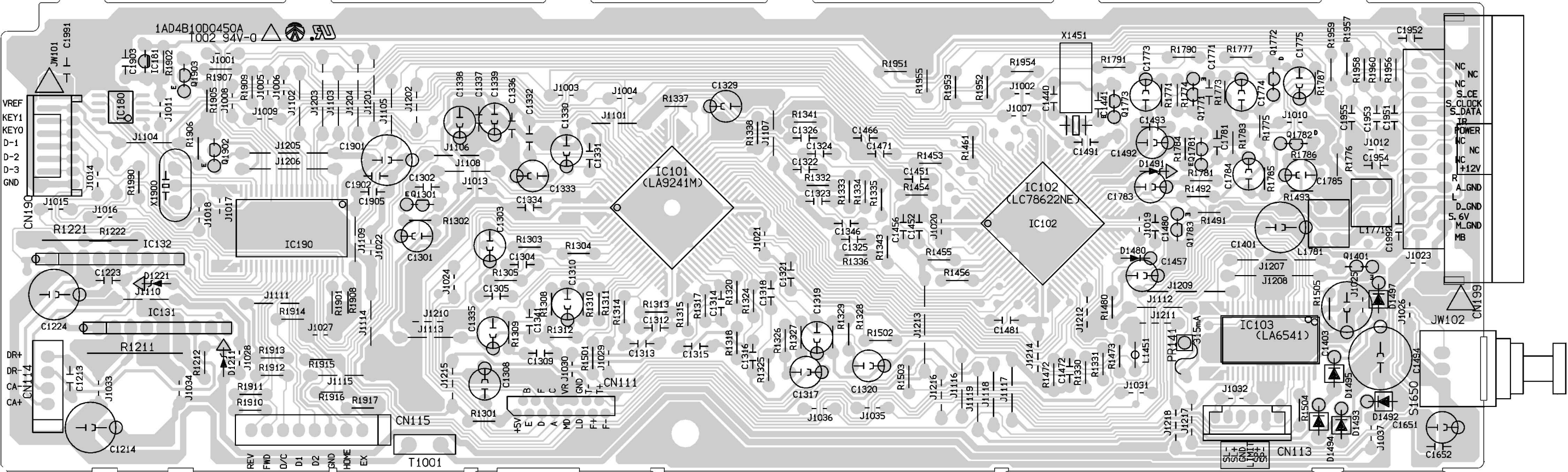
CD P.W.BOARD ASSY
