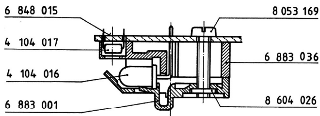
Teilschnitt A-B
