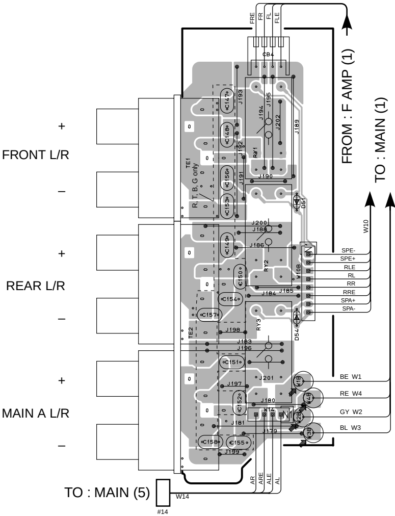
MAIN (4) P.C.B.
