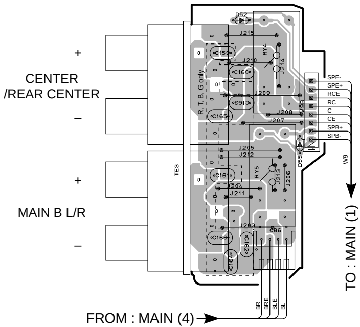
MAIN (5) P.C.B.
