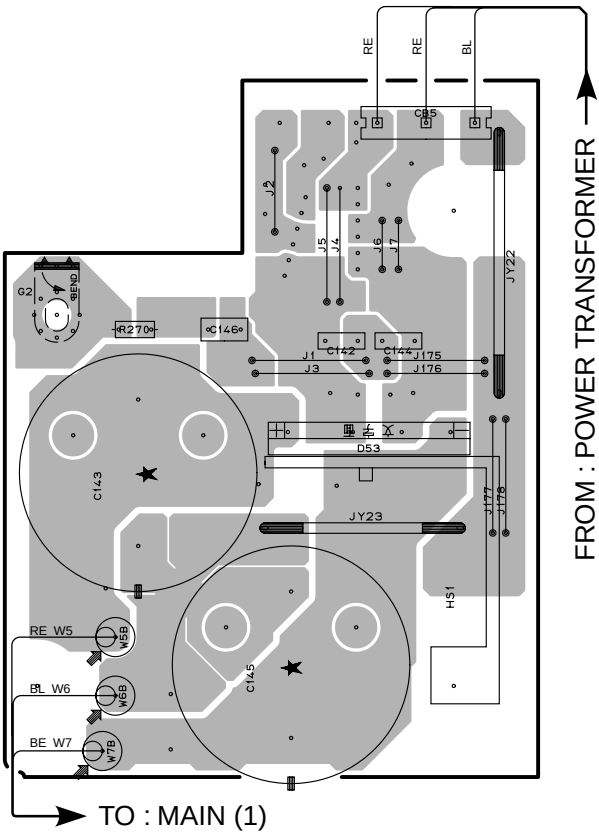
MAIN (2) P.C.B.
