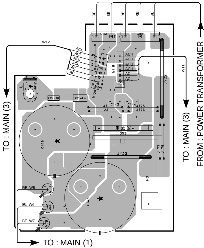
MAIN (2) P.C.B.
