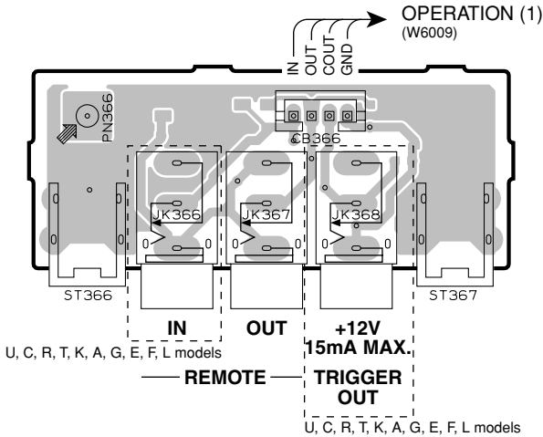
VIDEO (6) P.C.B. (Side A)
