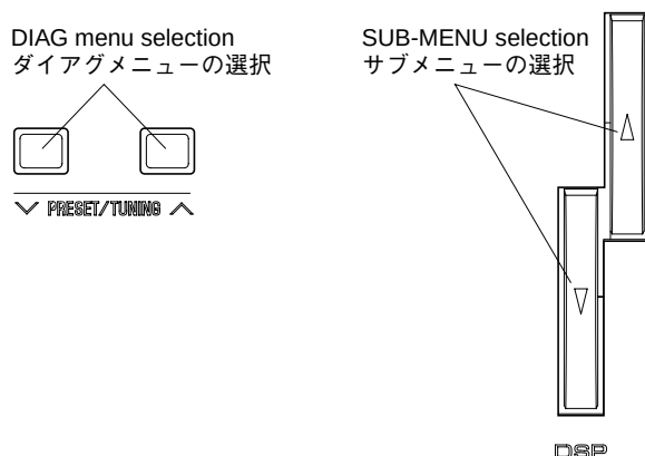
Keys of main unit / 本体キー
