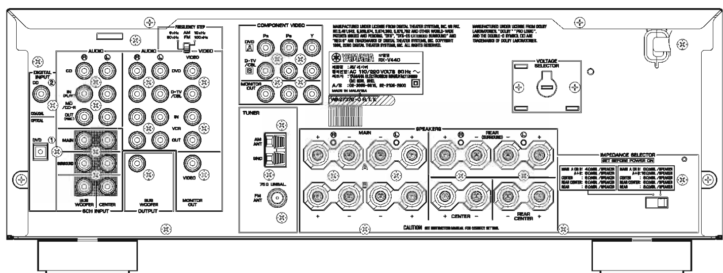
RX-V440 (K model)
