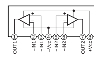
IC104 : NJM2068LD IC107-109 : MS220L Dual OP-Amp
